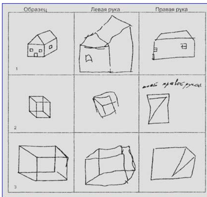
Рис. 18. Относительная неспособность левого полушария копировать геометрические фигуры. По Газзаниге.
