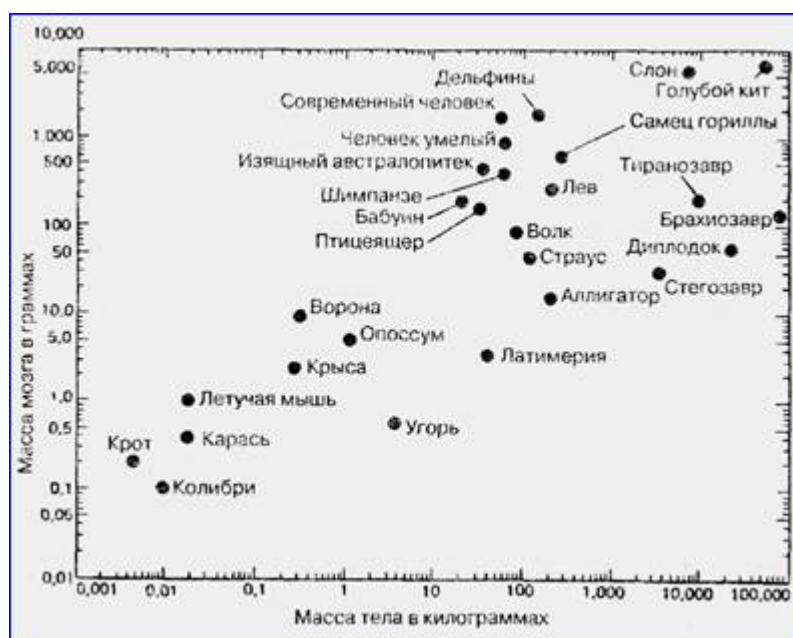
Рис. 5. Более подробное рассмотрение некоторых точек диаграммы, приведенной на рис. 4. Птицеящер — это страусоподобный динозавр, о котором говорится в этой книге.
