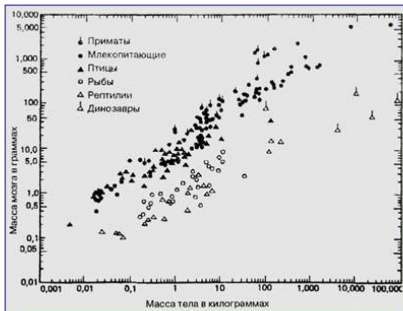
Рис. 4. Диаграмма, показывающая разброс величин «отношения массы мозга к массе тела» для приматов, млекопитающих, птиц, рыб, рептилий и динозавров
